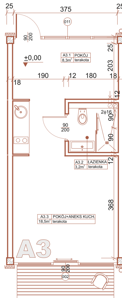
RZUT POZIOMY
